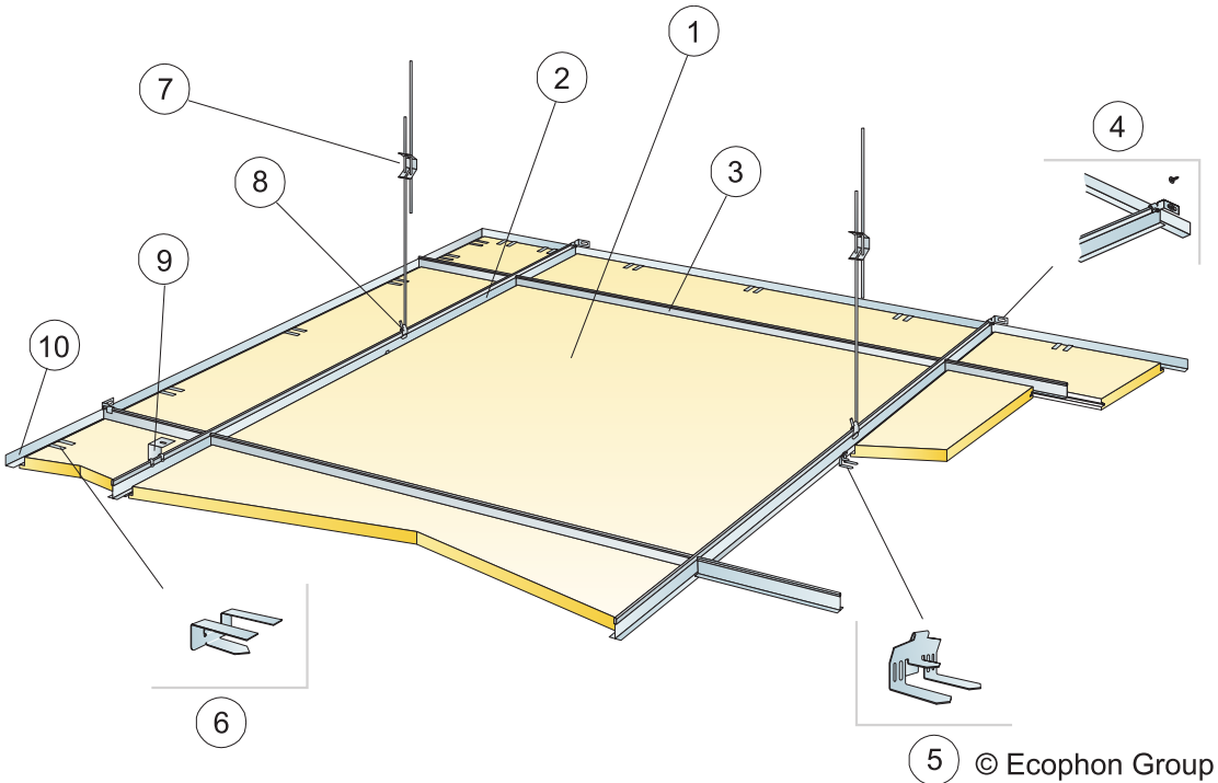
Diagrama de instalación (M203) para Ecophon Focus Dg 1200x1200 mm
