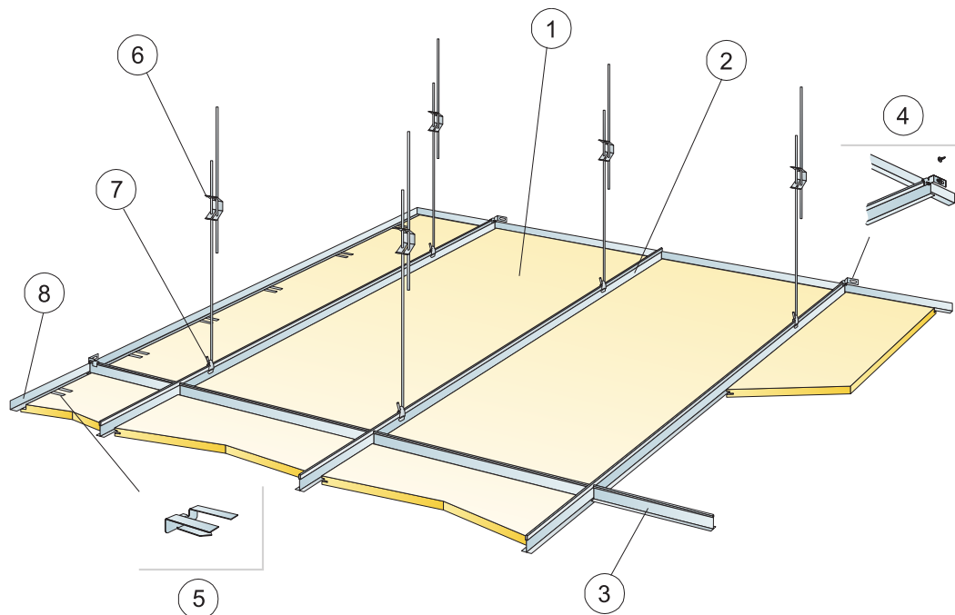
Diagrama de instalación (M204) para Ecophon Focus Dg XL
