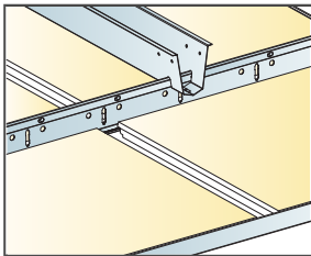
Instalación con perfil primario PL y galga
