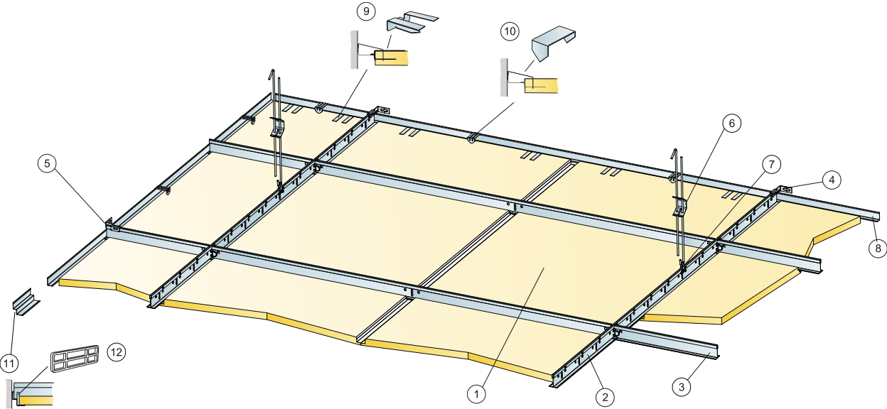
Diagrama de instalación (M583) para Ecophon Focus Ds 600x600, 1200x600 mm. Instalación suspendida.
