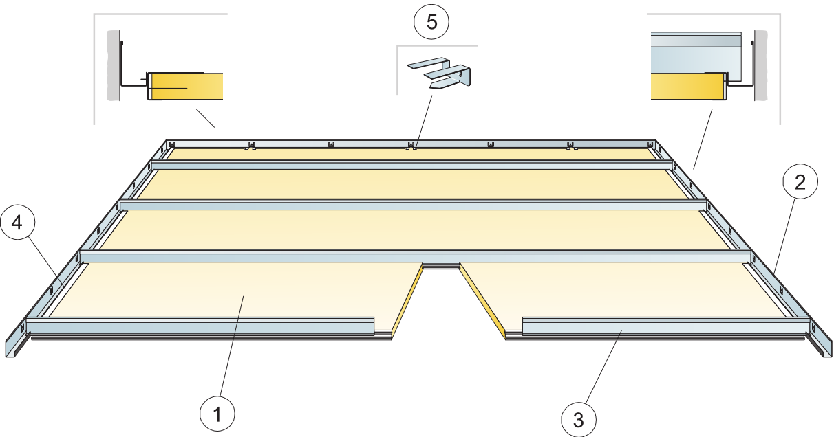
Diagrama de Instalación (M238) para Ecophon Focus Ds XL en pasillos.
