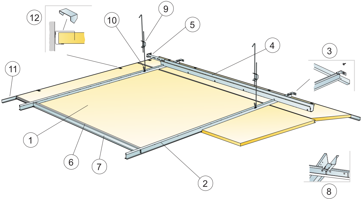
©Saint-Gobain Ecophon AB Diagrama de instalación (M582) para Ecophon Focus Ds 1200x1200 mm. Instalación suspendida
